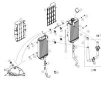
Radiador
